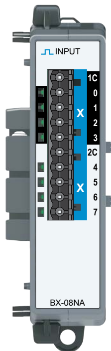
BX-08NA Input Module 8-pt, 120–240 VAC
