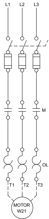
COMBINATION FUS / NON FUS. DISC.
